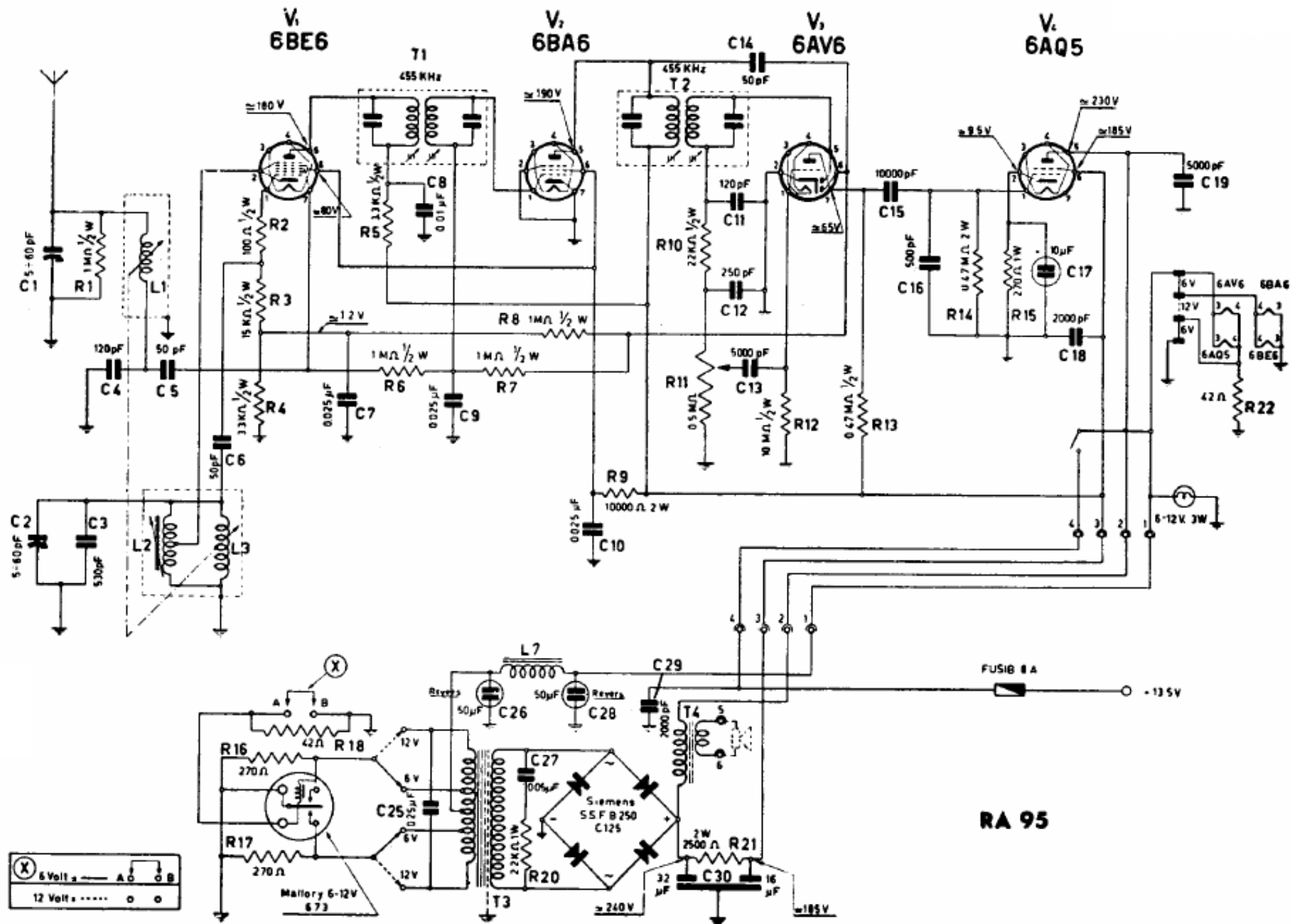
AUTOVOX - Mod. RA 95. Autoradio per la gamma onde medie, a permeabilità variabile. È costituito da due parti unite con un cavo a quattro conduttori. Media frequenza a 455 ke/s. Potenza d'uscita 1,5 watt. Consumo: 2,6 ampere a 13,5 volt.
